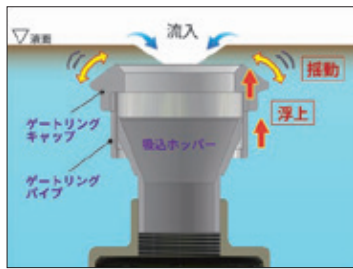
稼働時 ゲートリング部が浮上し揺動
