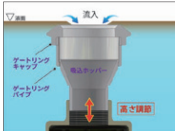
ねじ込みで高さを調節 (ゲートリング部は固定)
