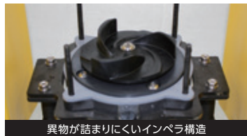
異物が詰まりにくいインペラ構造
