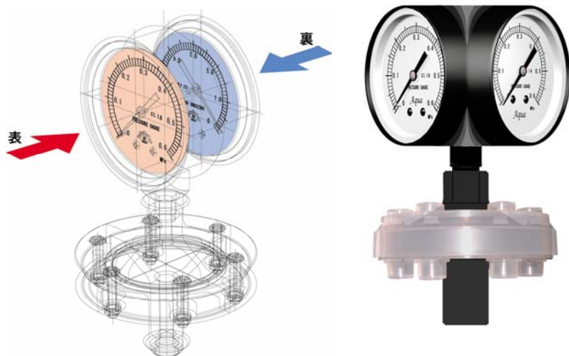
両面隔膜式圧力計イメージ図
